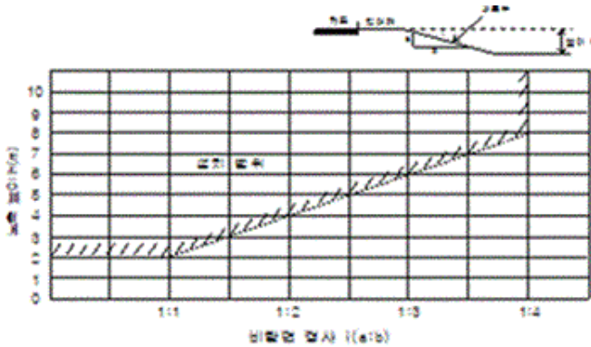
〈그림 2.4〉 비탈면 경사와 노측 높이와의 관계
