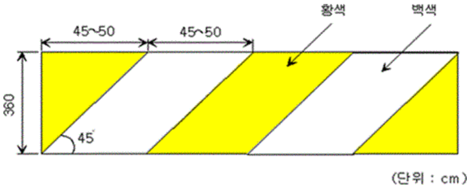
<그림 2.5> 과속방지턱의 표면 도색 2.5 설치
