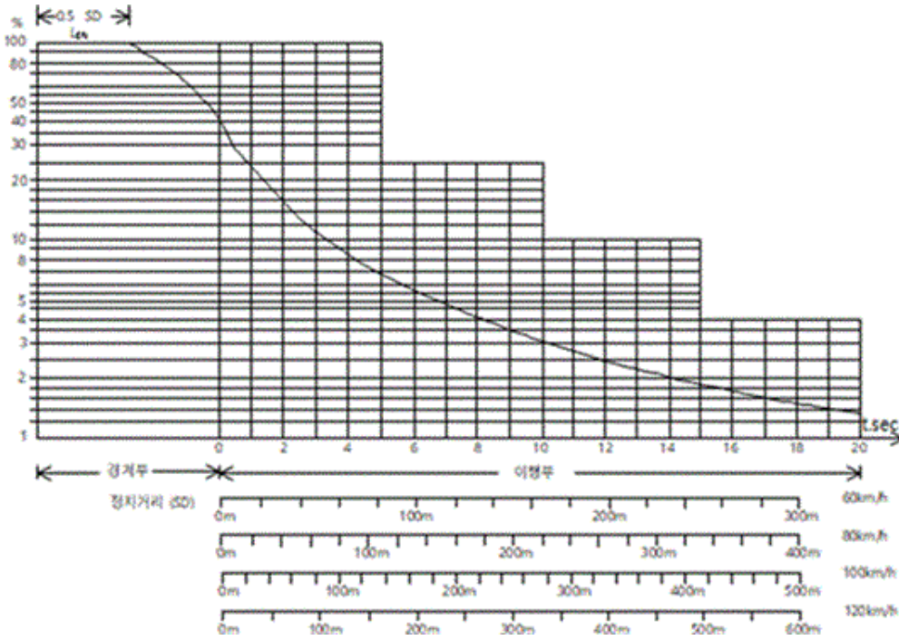
<그림 6.4> 터널 입구부의 노면휘도
